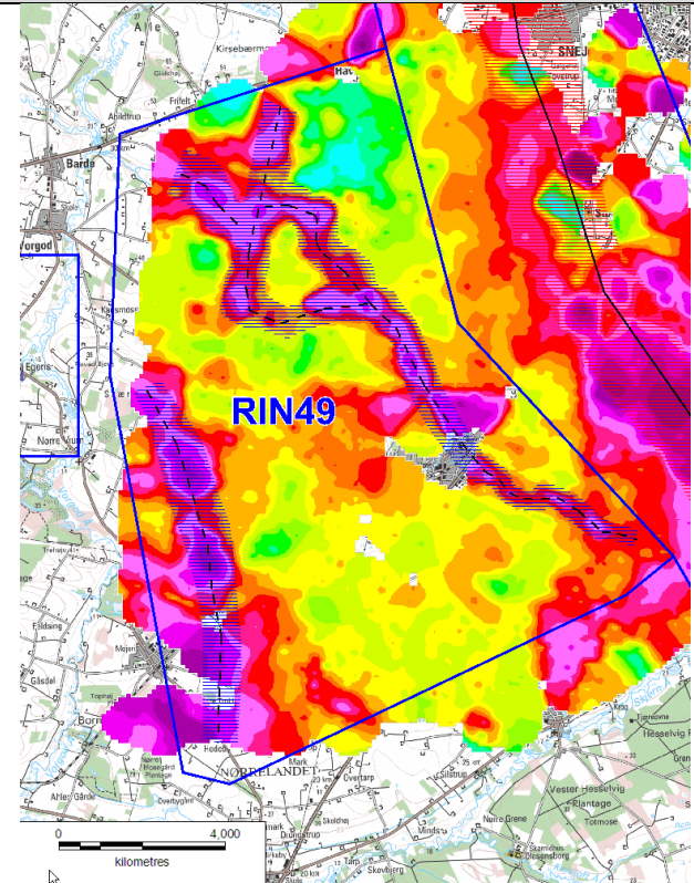
Figur 2: TEM middelmodstandskort kote +5 m:
